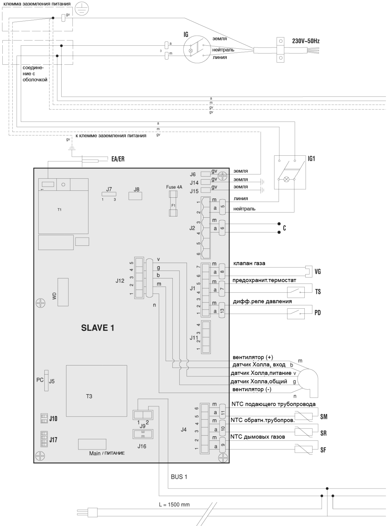
Шина с разъемом «папа» для соединения с другим котлом модели 100S
